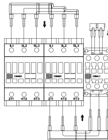
Barras para arranque estrella-triángulo
